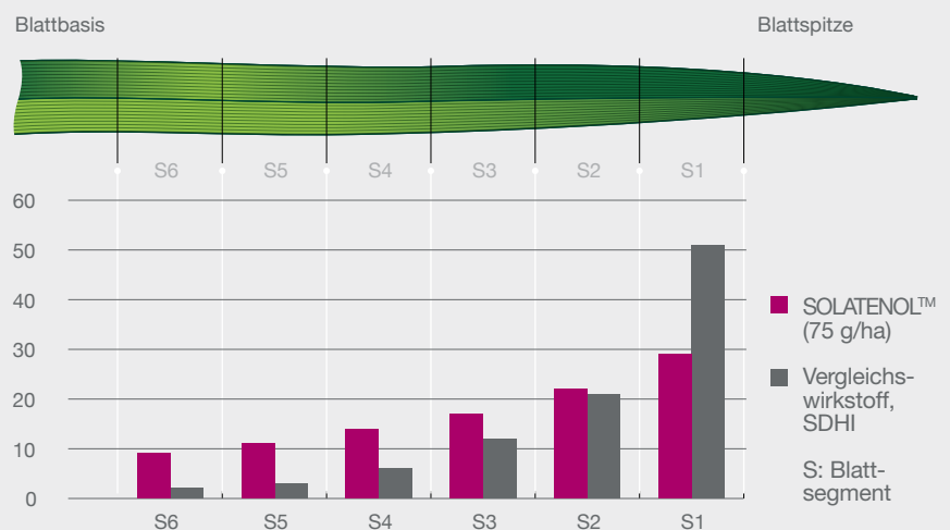
Wirkstoffverteilung (%), 14 Tage nach Applikation
